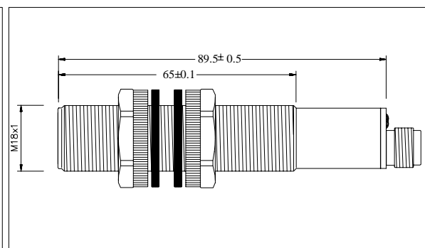
Abmessungen/ Dimensions mm
